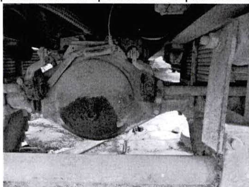
Fig. 6, 7 diferencial en mal estado conjunto de eje cardan
