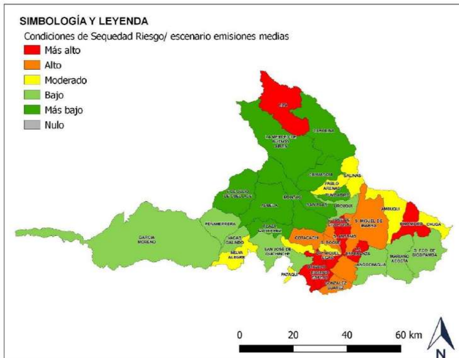
Mapa 44. Riesgo de cultivos ante condiciones de sequedad, escenario de emisiones medias.
