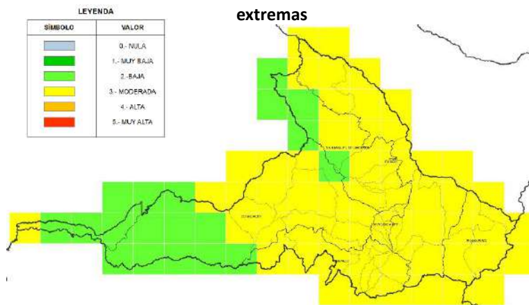
Mapa 34. Nivel de amenaza para las lluvias intensas, según la tendencia de aumento del número de días al año con lluvias extremas
