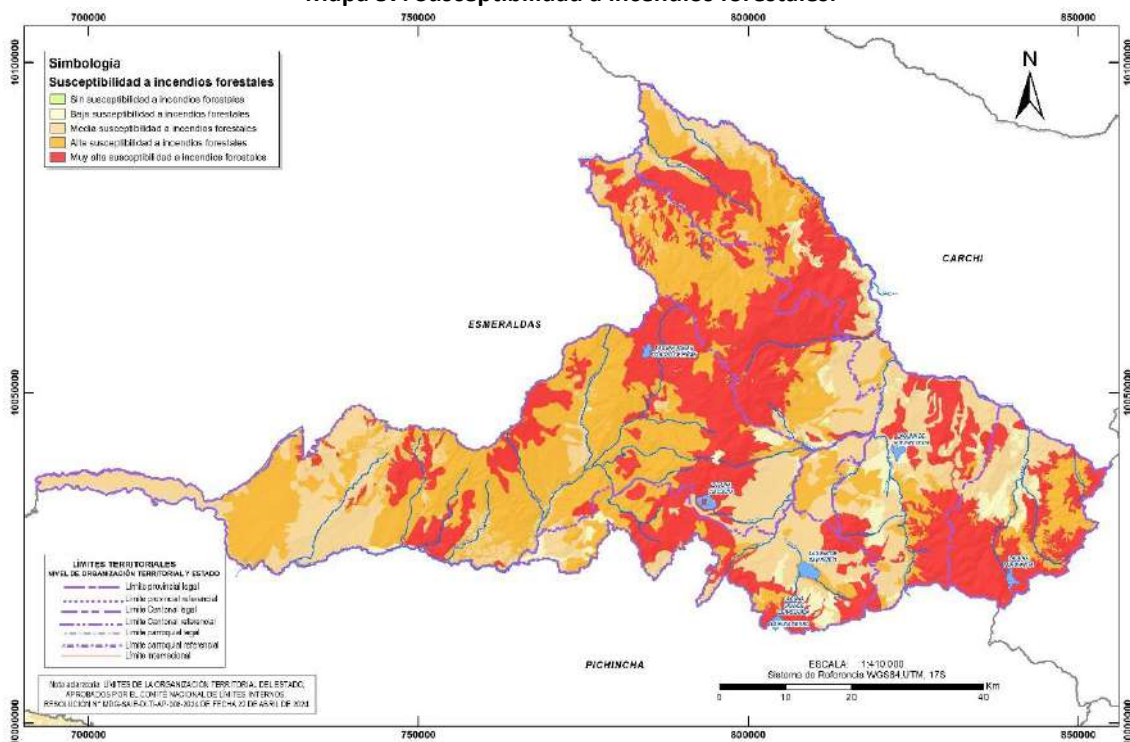
Mapa 57. Susceptibilidad a incendios forestales.
