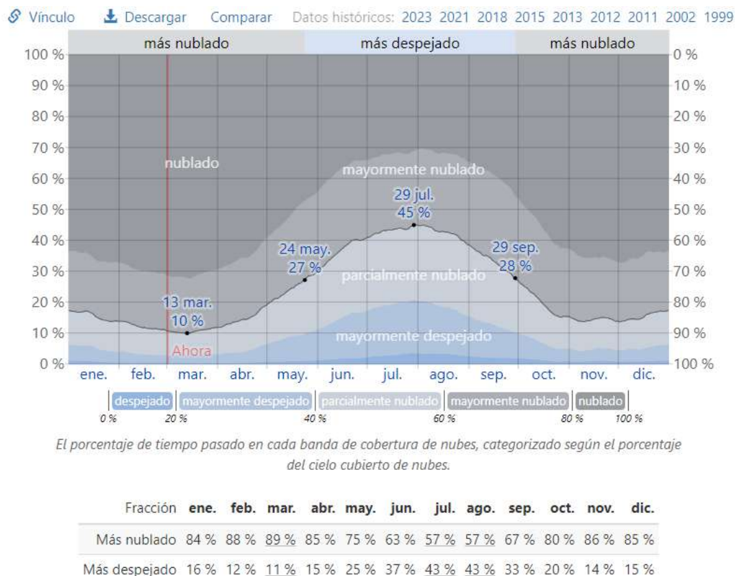
Figura 5. Categorías de nubosidad en Ibarra.
