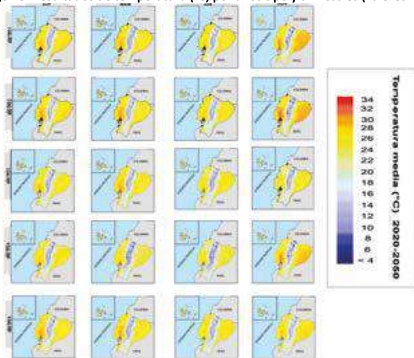
Imagen 8. Resultados de temperatura (°C) por años tipo y trimestres (valores netos).
