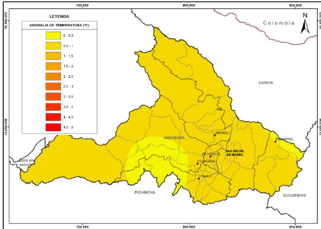
Mapa 31. Cambio de la temperatura media (°C) proyectado bajo el escenario RCP 4.5 para el periodo 2016-2040, con relación al periodo histórico 1981-2015.
