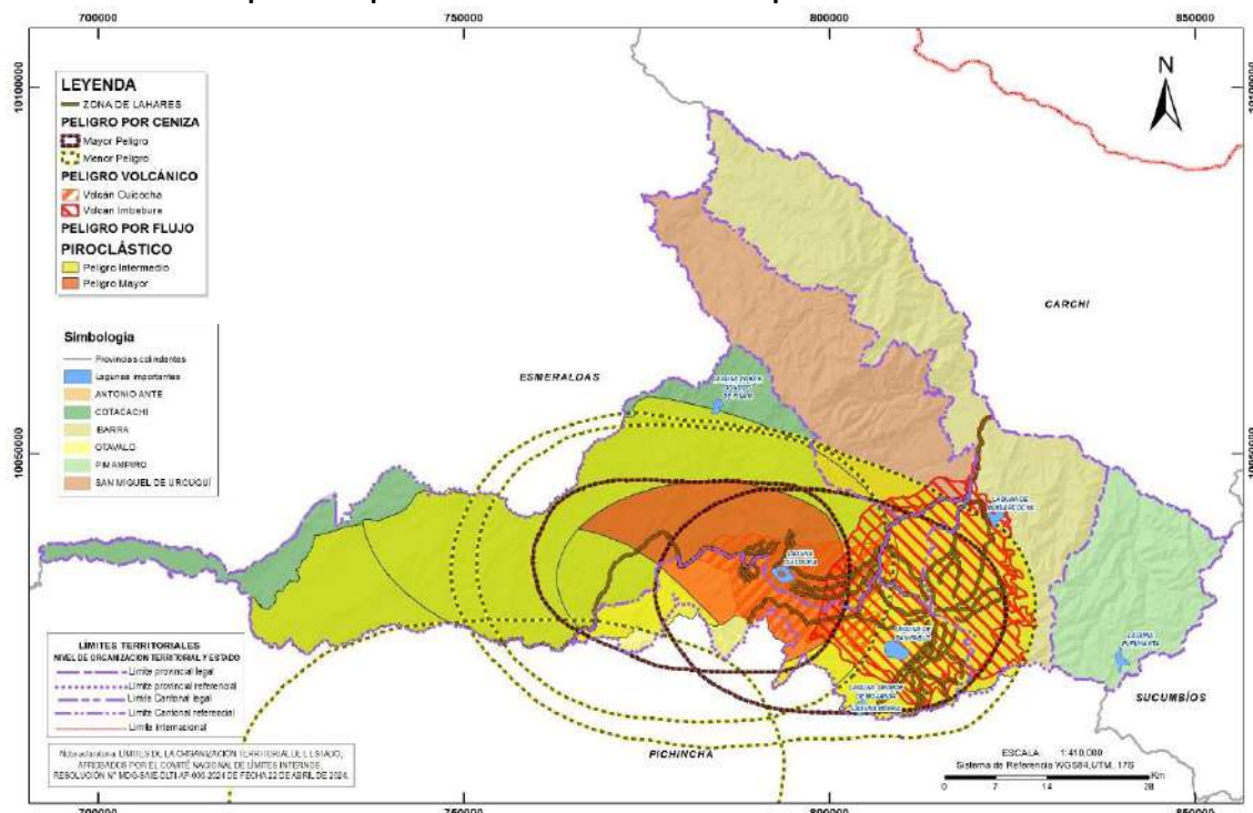
Mapa 20. Mapa de amenazas volcánicas de la provincia de Imbabura.
