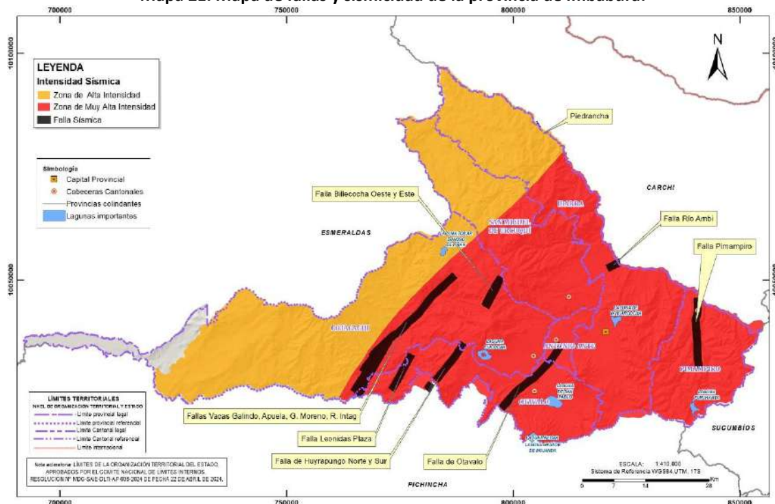
Mapa 21. Mapa de fallas y sismicidad de la provincia de Imbabura.
