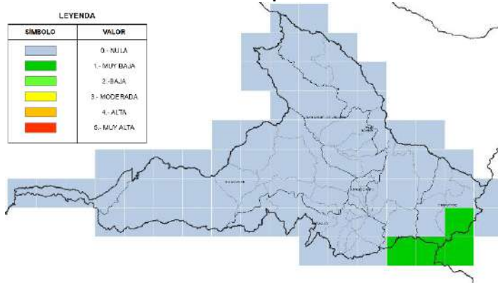
Mapa 32. Nivel de amenaza bajo los escenarios de cambio climático RCP 4.5 en el periodo 2016-2040
