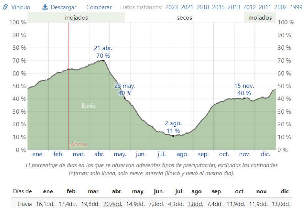
Figura 6. Probabilidad diaria de precipitación en Ibarra.
